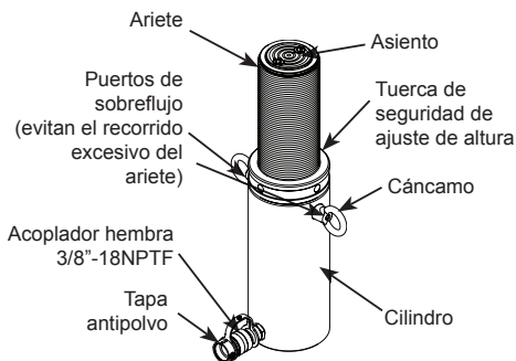
Figura 1: Componentes habituales del cilindro
